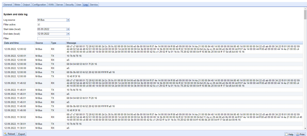
Abbildung 28: Tab Log
