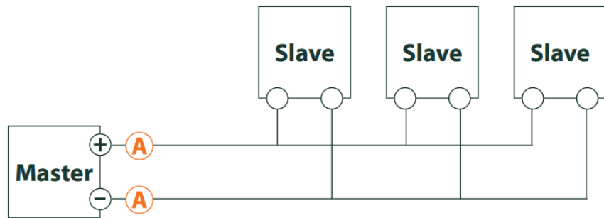
Abbildung 33: Fehlersuche beim M-Bus durch Messung mit Multimeter
