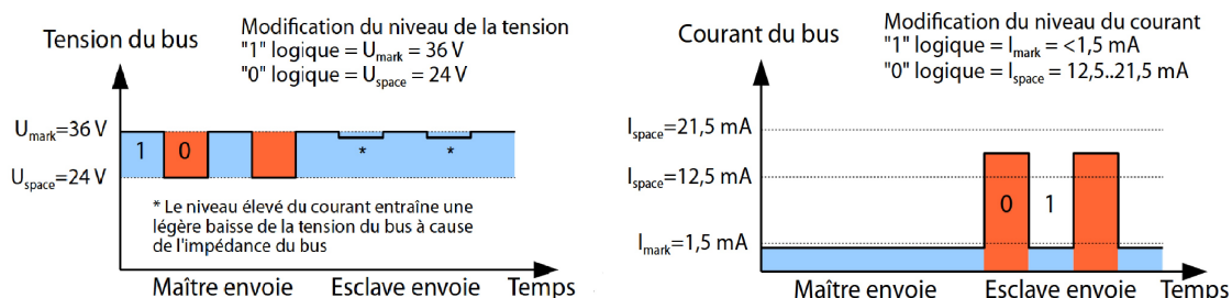
Figure 2 – Signalisation sur le M-Bus
